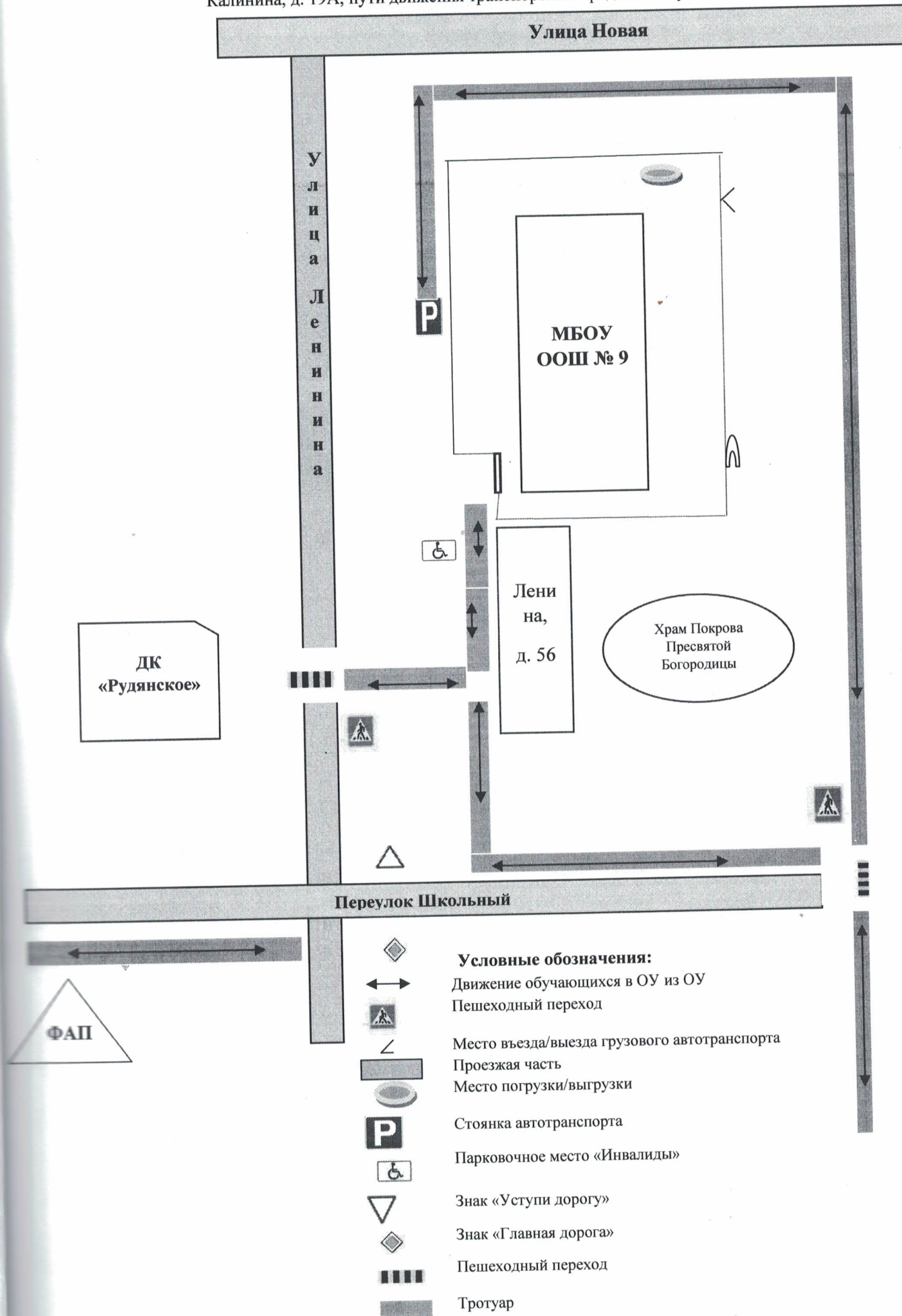
Схема № 1. Район расположения образовательного учреждения МБОУ ООШ № 9, с. Рудянское, ул. Калинина, д. 19А, пути движения транспортных средств и обучающихся
