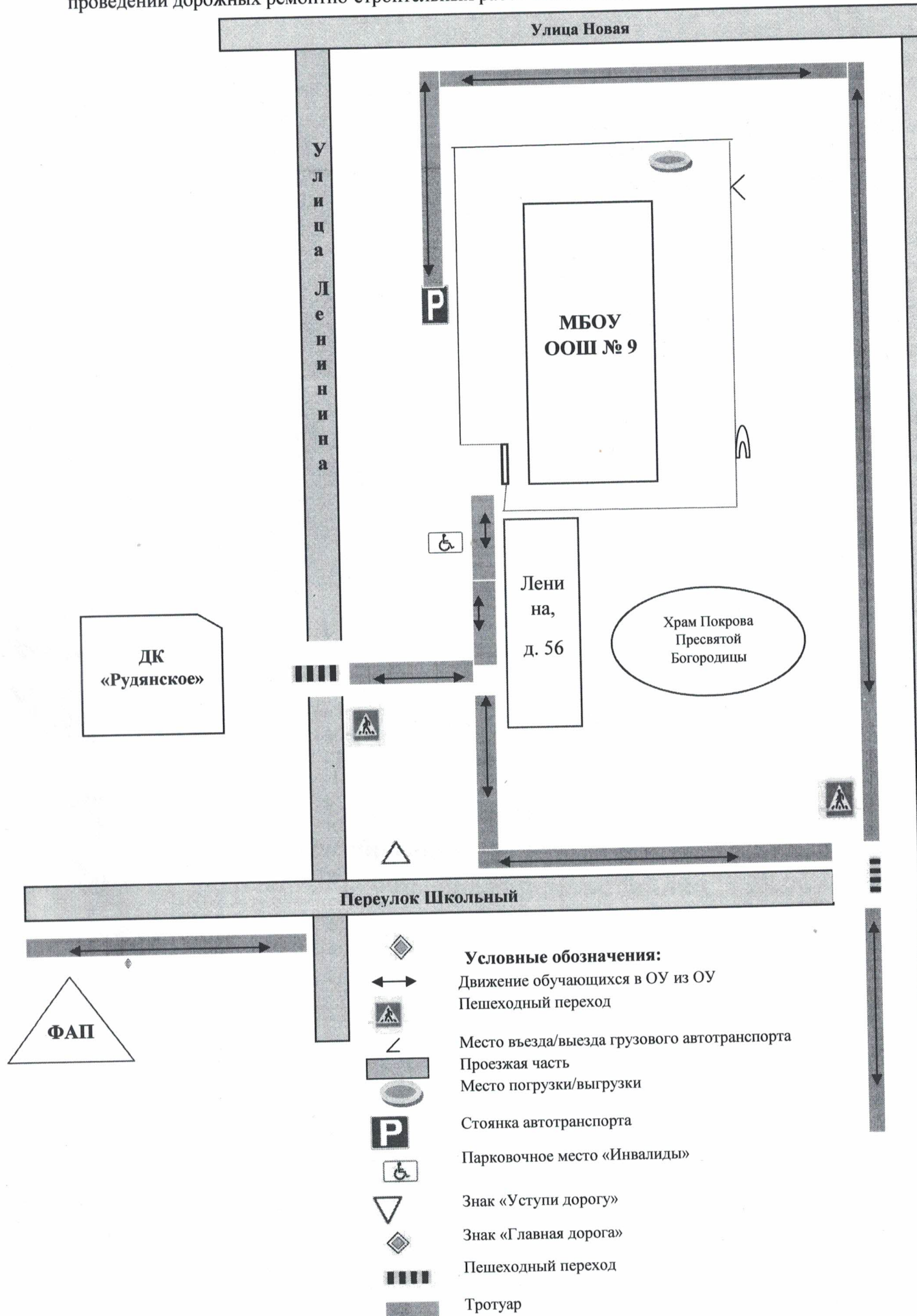
Схема № 5. План-схема пути движения транспортных средств и обучающихся при проведении дорожных ремонтно-строительных работ вблизи МБОУ ООШ № 9.
