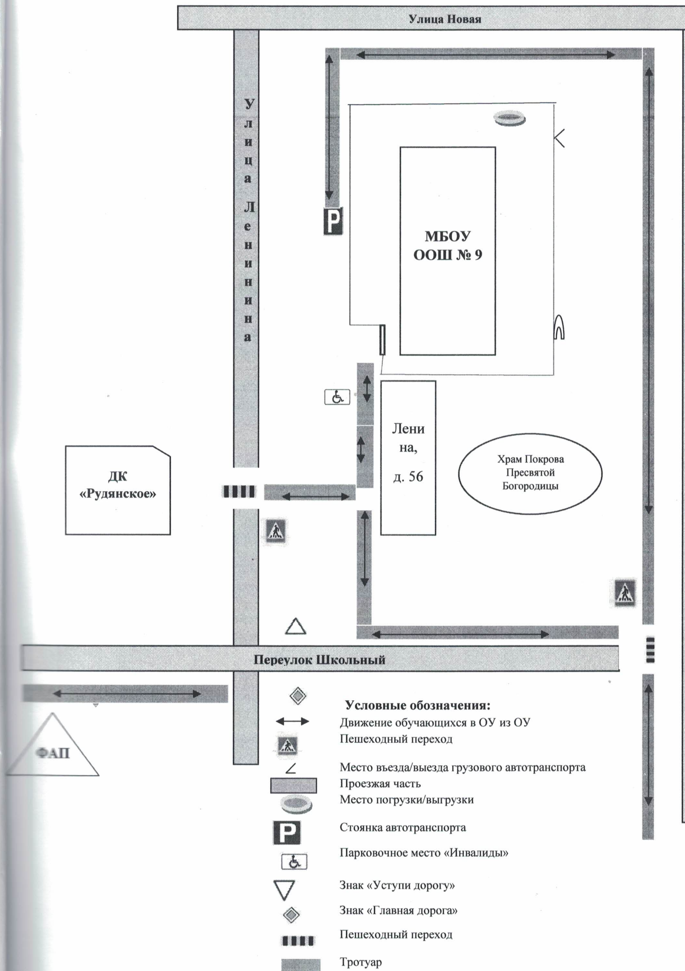
Схема № 2. Организации дорожного движения в непосредственной близости от МБОУ ООШ № 9 размещением соответствующих технических средств организации дорожного движения
